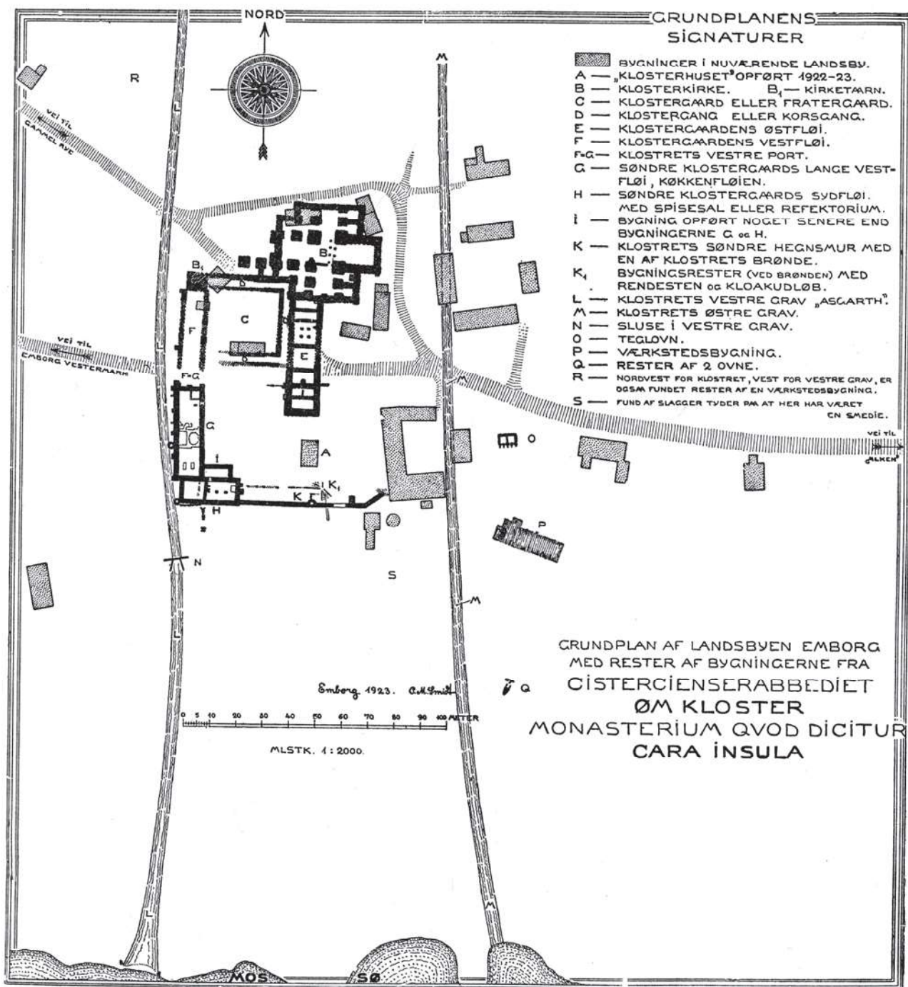
Fig. 1.5. C.M. Smidts oversigtsplan indtegnet på et kort over landsbyen Emborg. Da grundplanen blev tegnet, var ruinparken stadig delt i to af de tværgående veje, og den nordlige del af kirken ej heller frilagt endnu. Opmåling: C.M. Smidt 1923.
