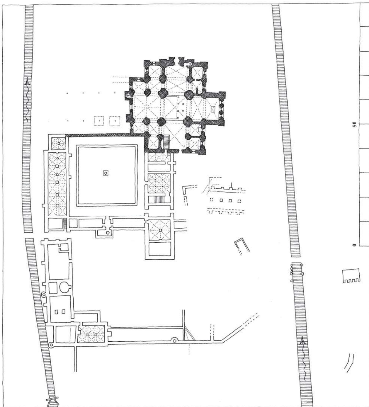
Fig. 1.9. Plan fra Danmarks Kirker. I forhold til den skematiske plan fra udgravningerne i 1970'erne har man her forsøgt en nuanceret rekonstruktion med en række tolkninger af pillernes udformning m.v. Planen er specielt udarbejdet til illustration af mulige forhold i kirken, der derfor er skraveret. Tegning: Kjeld de Fine Licht, Nationalmuseet 1992.
